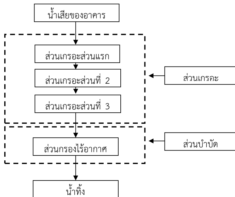
รูปที่ ก-1 แสดงรูปแบบของระบบบำบัดน้ำเสียสำหรับอาคารใช้อู่อาศัย
